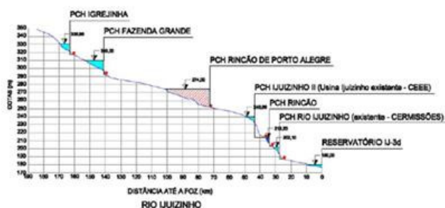
Figura 23: Localização da PCH Rincão
