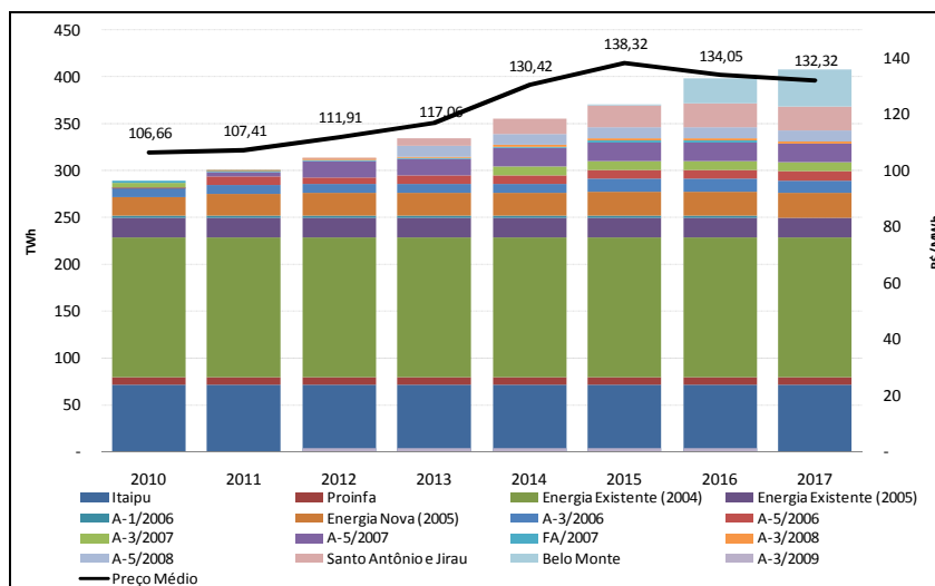
Figura 18: Curva de preço do ACR (R$/MWh)
