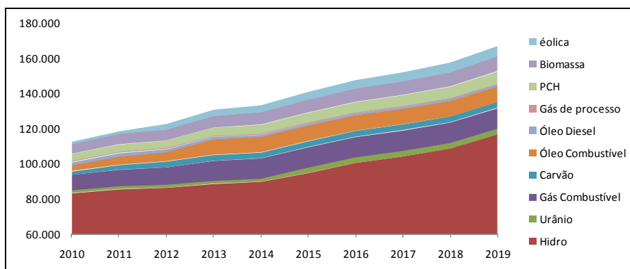
Figura 13: Evolução da capacidade instalada de geração (MW)
