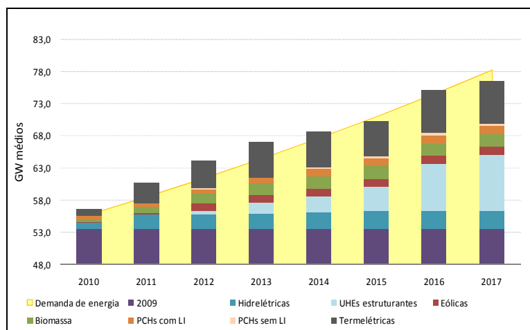
Figura 12: Balanço Energético (GW médios - 2010)
