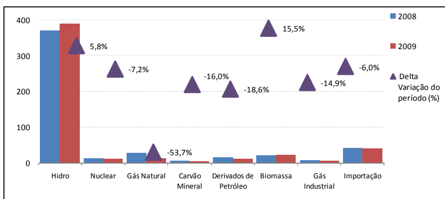
Figura 4 - Oferta Interna de Energia Elétrica (OIEE) – 2009 (TWh)
