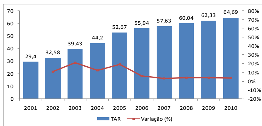
Figura 20: Histórico da TAR (R$/MWh)
