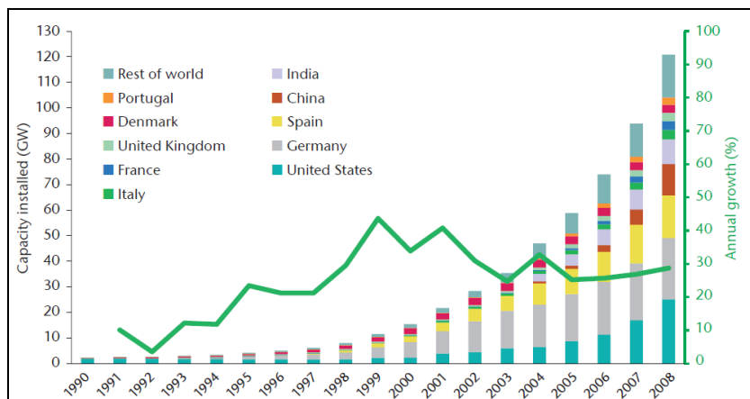
Figura 8: Crescimento da potencia instalada por fonte eólica
