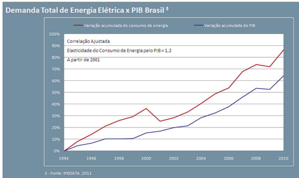
Figura 11: Demanda Total de Energia x PIB Brasil
